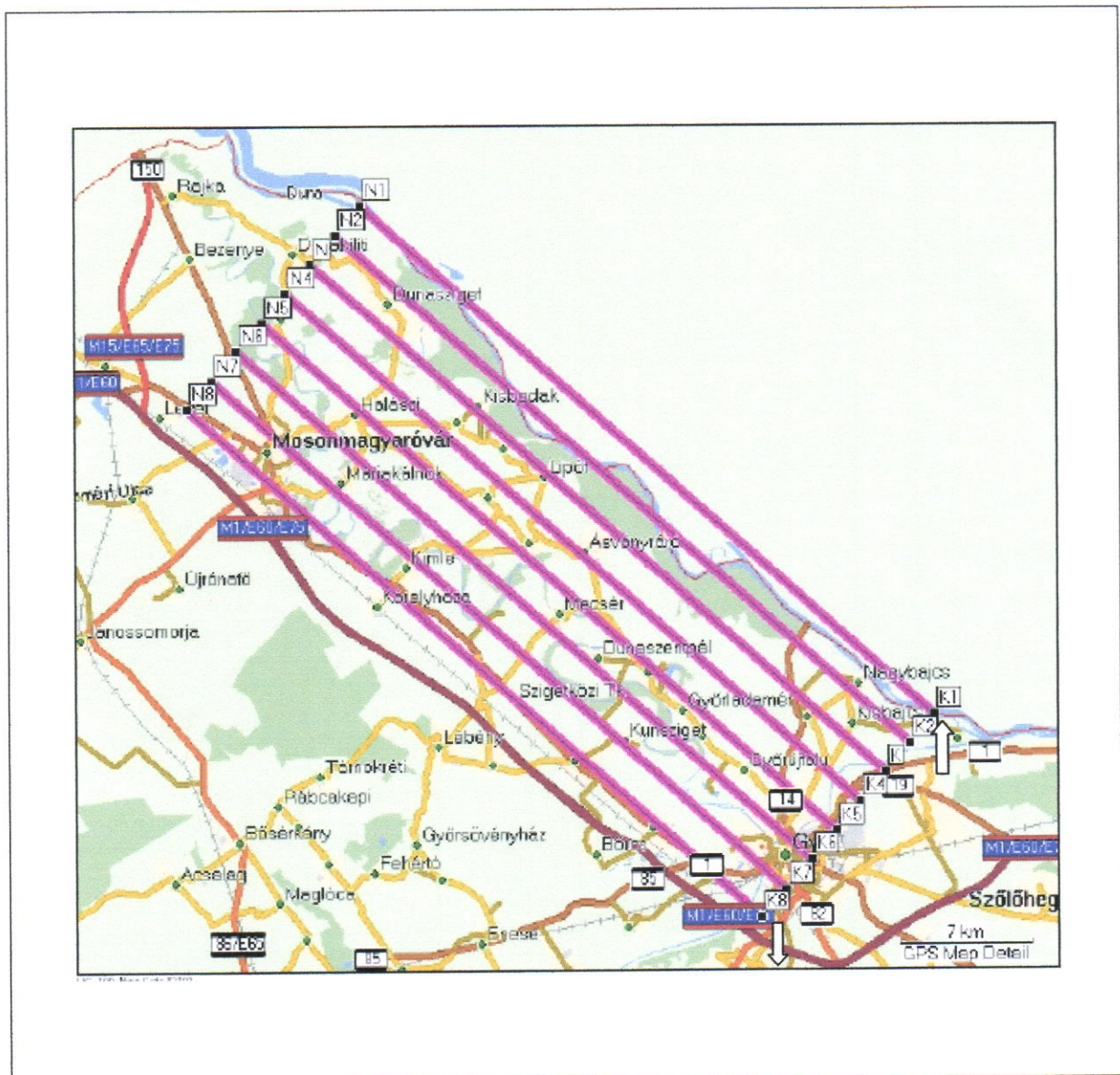
1. ábra A 2006. augusztusra tervezett szigetközi légifelvételzés GPS alapú repülési tervének vázlata
